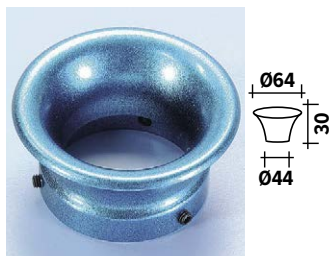
203.1501 Ø44
